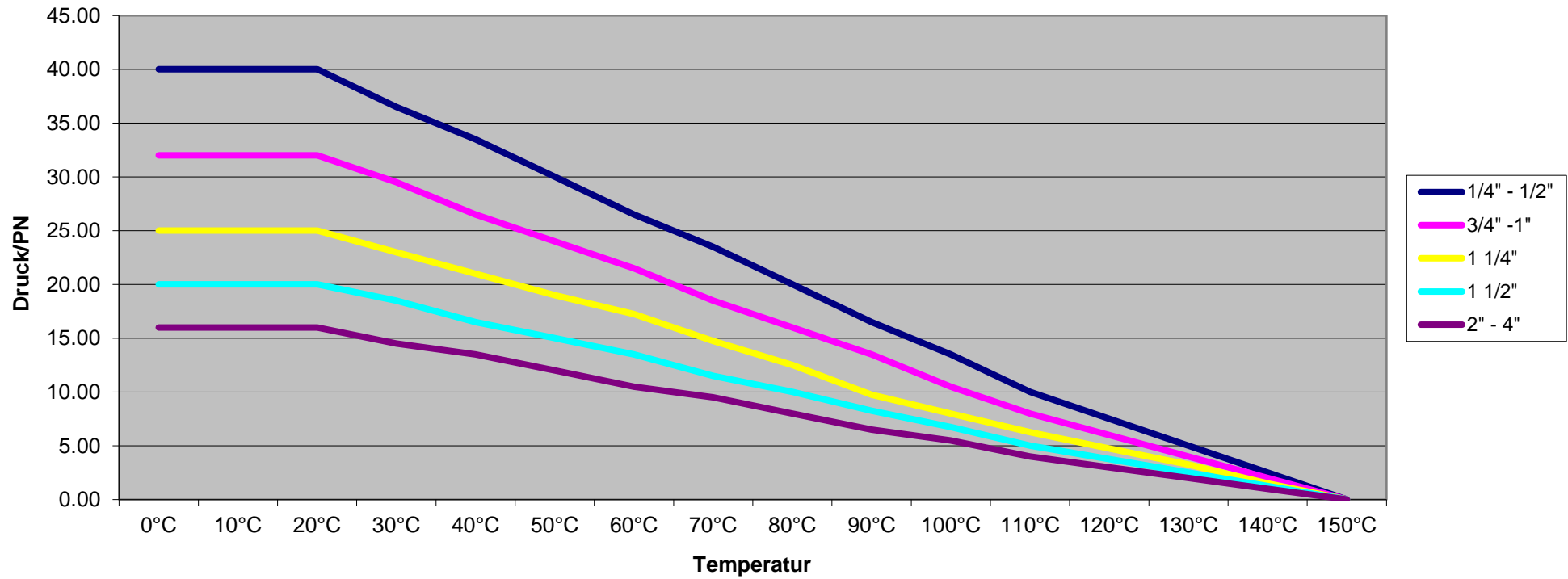
Druck-/Temperaturdiagramm zu Kugelhähne Art.-Nr.: 600, 606, 610, 616 und 756
